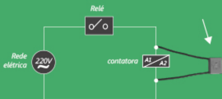
Ligação em contadora
