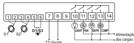
Imagen III - Conexión 12 Vac/dc
