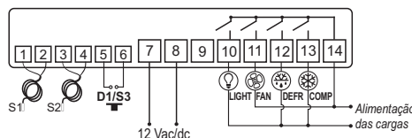
Imagen III - Conexión 12 Vac/dc
