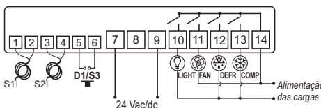
Imagen IV - Conexión 24 Vac/dc
