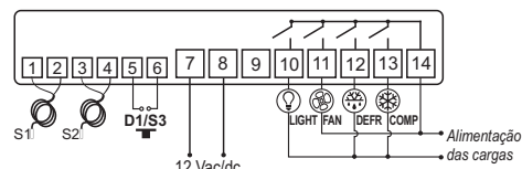
Imagen III - Conexión 12 Vac/dc
