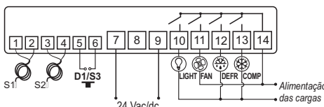
Imagen IV - Conexión 24 Vac/dc
