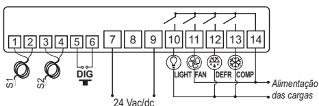
Imagen IV - Conexión 24 Vac/dc
