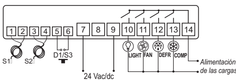
Imagem IV - Conexión 24 Vac/dc
