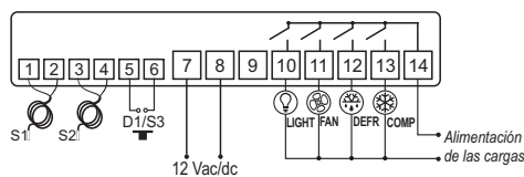
Imagem III - Conexión 12 Vac/dc
