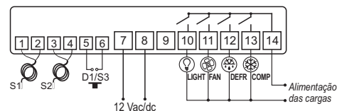
Imagem III - Conexão 12 Vac/dc
