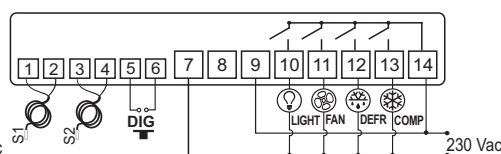
Imagem II - Conexão 230 Vac
