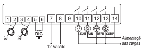
Imagem III - Conexão 12 Vac/dc
