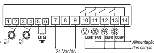
Imagem IV - Conexão 24 Vac/dc
