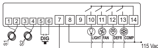
Imagem I - Conexão 115 Vac
