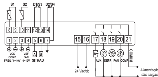
Imagem III - Conexão 24 Vac/dc
