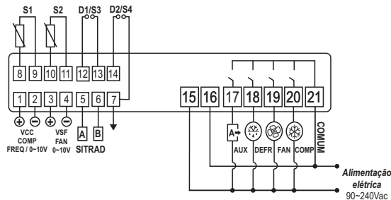
Imagem II - Conexão 12 Vac/dc
