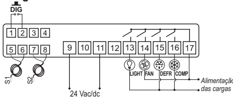
Imagem IV - Conexão 24 Vac/dc
