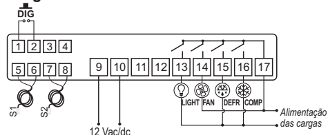
Imagem III - Conexão 12 Vac/dc
