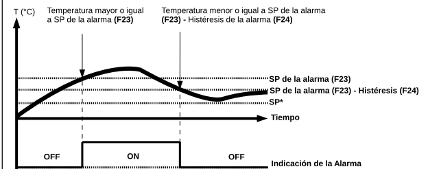
Figura 1 - Alarma superior absoluta
