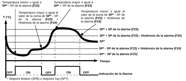
Figura 3 - Alarma extra banda
