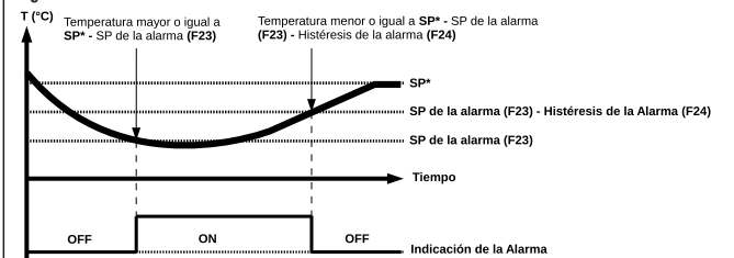
Figura 2 - Alarma inferior relativa
